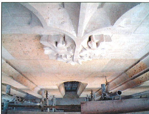
Istočni zid sjevernog tornja nad krovom katedrale
