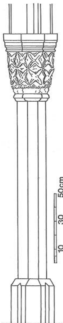
Sl. 6. Kapela sv. Stjepana Prvomučenika, polustup u jugoistočnom kutu kapele (Crtež: kao slika 5.)
