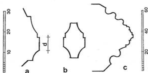
Sl. 11 Kapela sv. Stjepana Prvomučenika, neke profilacije iz kapele: a. Prozori u južnom zidu; b. Ulomak šprilja prozora, nađen prigodom iskopa za instalacije pred kapelom; c. Profilacija velike rozete u zapadnom zidu (Crtao: Z. Horvat)
