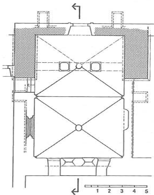
Sl. 2. Kapela sv. Stjepana Prvomučenika u nadbiskupskoj palači: ucrtani su veliki ranogotički kontrafori te spojni zid među njima (označeni rasterom). Zidovi kapele su naknadno podebljavani. Polovica sjeverna dijela svoda bila je srušena zbog gradnje hodnika na prvom katu barokne palače u 18. st.
