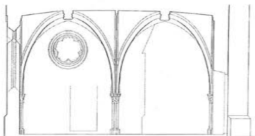
Sl. 4. Kapela sv. Stjepana Prvomučenika, presjek i pogled na zapadni zid; svod je nacrtan bez kasnijeg ubacivanja hodnika I. kata barokne palače. Malo desno, ispod rozete nađeni su tragovi prvotna ulaza u kapelu (Crtao: Ivan Tenšek)
