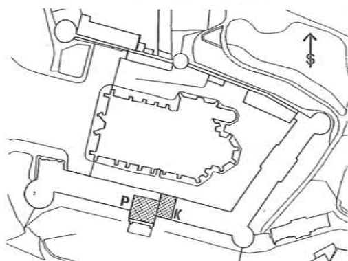
Sl. 1. Zagreb, situacija katedrale i utvrda oko nje. Dolje, na južnoj strani, nacrtana je nadbiskupska palača i ucrtana kapela sv. Stjepana Prvomučenika (K) te srednjovjekovna biskupska palača (P)
