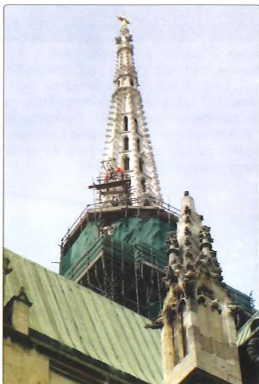
Na vrhu skele sjevernog zvonika montiraju se i premještaju konzole za dizalicu, kojom se kamen sa radne platforme treće galerije, na visini 65 m, podiže do mjesta ugradnje, na visinama do 75 m.
