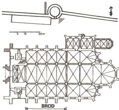
Situacija katedrale i sjeverne kule: trokut pokazuje mjesto na kuli gdje je ugrađen naš ulomak rebra (Crtao Z. Horvat)
